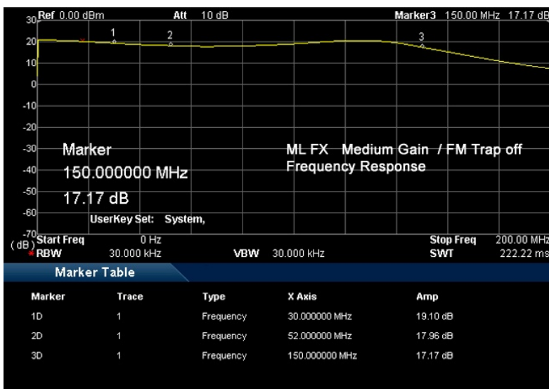
MegaLoop FX標準特性(利得:ミドル、FMトラップOFF)
